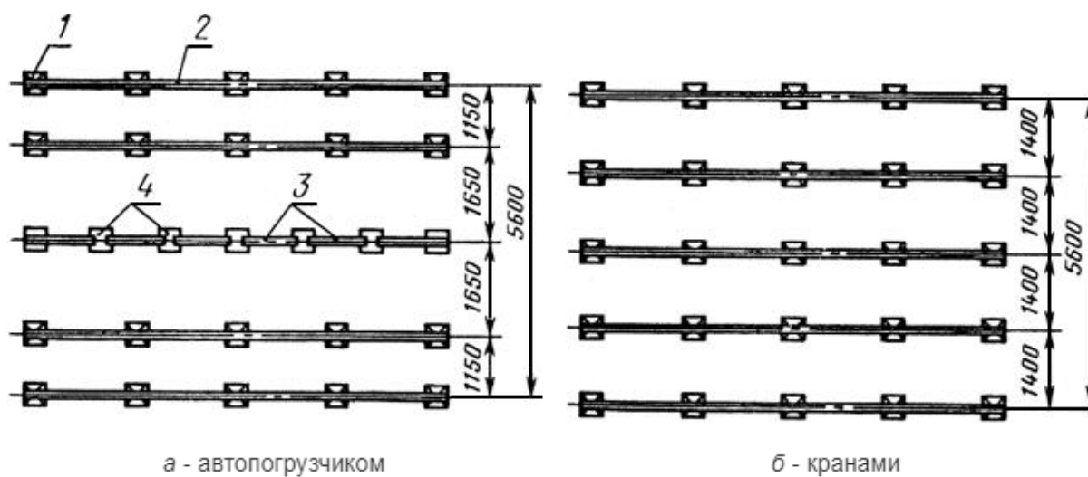
"Черт. 4. Схема подштабельных фундаментов для укладки пакетных штабелей"
